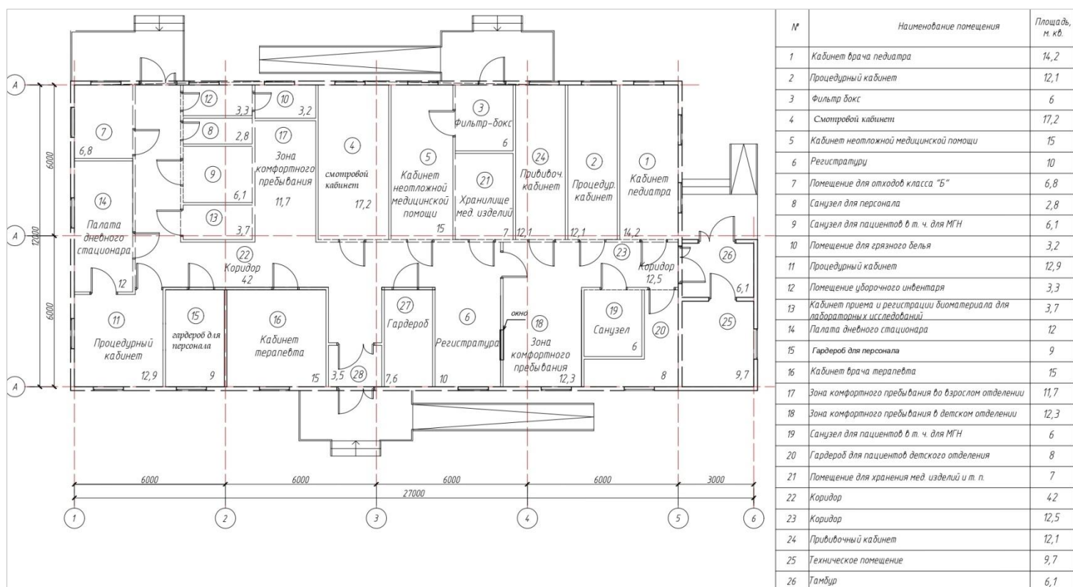
Рис.1. - План здания с экспликацией помещений
